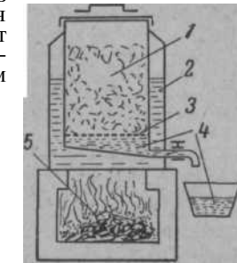
Рис. 2. Водяная воскотопка: 1 — сушь; 2 — вола; 3 — решетка; 4 — воск; 5 — топка.
