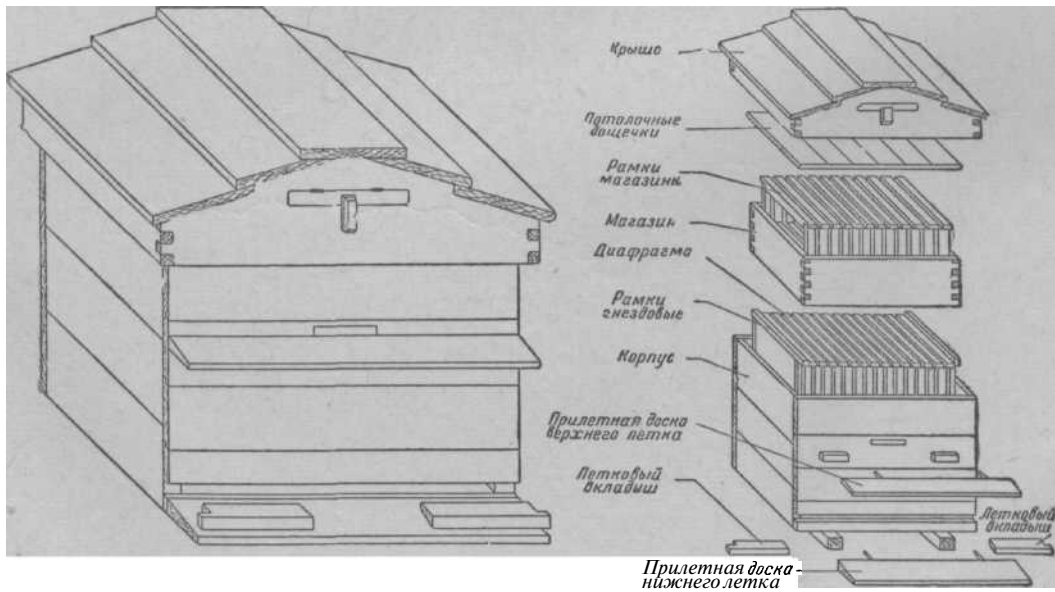
Рис. 4. Двухстенный улей на 14 рамок (общий вид и детали устройства).
