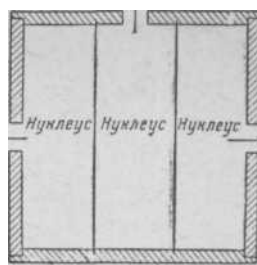
Рис. 3. Схема использования корпуса стандартного улья для трех нуклеусов.
