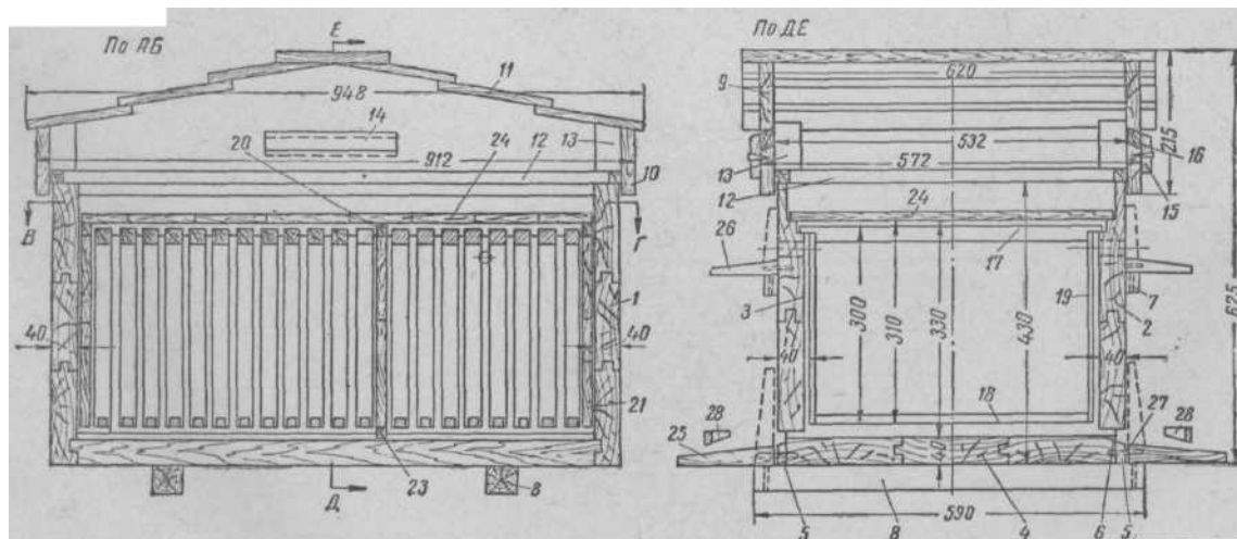
Рис. 6. Размеры улья-лежака.
