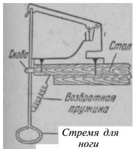
Рис. 3. Схема работы дырокола от ножной педали.
