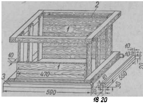
Рис. 1. Каркас корпуса соломенного улья в полусобранном виде: 1 — передняя и задняя стенки, каждая из сплошного настила досечек, расположенных в горизонтальном направлении; 2 — фальцы для навешивания рамок; 3 — наружные планты, образующие вокруг корпуса борт (глубиной 10 мм), необходимый для соединения корпуса с дном и корпуса с корпусом.
