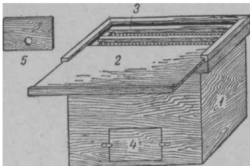
Рис. 2. Ящик-роевня: 1 — корпус; 2 — выдвигная крышка; 3 — рамки; 4 — глухая отъемная дверка (применяется при переноске расплода, перевозке роев и пчелиных семей); 5 — ручка; 6 — дверка с летковым отверстием.
