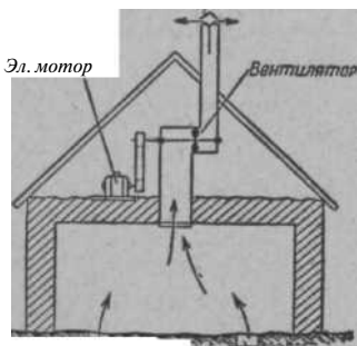
Приточные каналы
