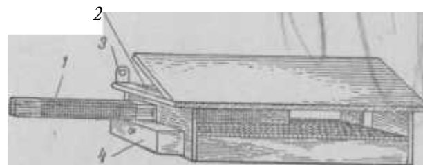
Рис. 36. Общий вид пыльцеуловителя: 1 — выдвижная рамка-решетка; 2 — боковой проход для вылета пчел из улья; 3 — петля для подвешивания прибора к летку улья; 4 — выдвижной ящик для обножки
